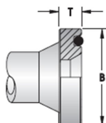
SAE O'RING FLANGE
